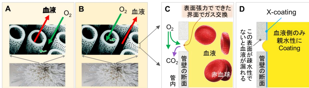
図 2. ホロファイバーの束(下パネル)とその拡大図(上パネル)及びガス交換の仕組み。 A: 初期の人工肺では、ホロファイバーの管腔内に血液を流す方式だったために層流によるガス交換性能の限界があった。 B: 野川さんは逆転の発想で見事にこの問題を解決した。 C: 細管壁に開けられた多数の細孔を通してガス交換(酸素 O_2 添加)が行われる。図では 1 個の細孔部を拡大表示している。細孔表面が疎水性であるために、水の表面張力によって、あたかも水分子の薄い膜で界面が覆われたかのように、水が漏れないと同時にその界面から O_2 が浸透し、赤血球中のヘモグロビンに結合して全身に運ばれる。 D: プラスティック表面は血球や血液成分にダメージを与えやすいので、PMEA [poly(2-methoxyethyl acrylate)] 等のポリマーで被覆し、悪影響が出ないように工夫されている。このとき 如何にして 必要な面のみをコーティングするかが要となる。
